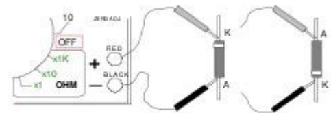
MENGUJI KERUSAKAN DIODA
