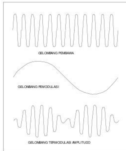
MODULASI AMPLITUDO
