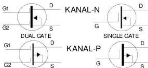
SYMBOL MOSFET
