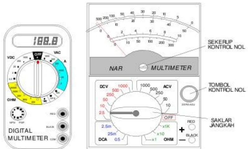
AVOMETER
