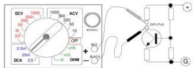
PENGUKURAN ARUS DC
