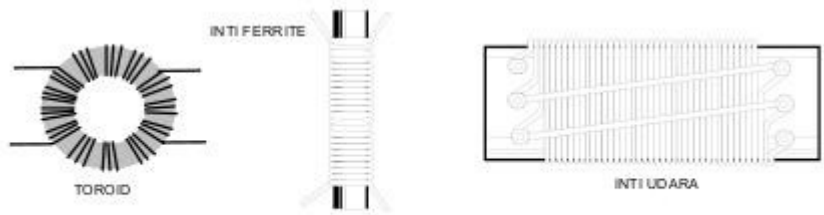
BERBAGAI MACAM BALUN
