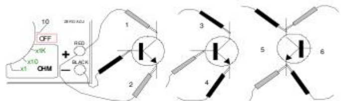
MENGUJI TRANSISTOR
