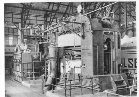
7. Zenderaal te Malabar. Gezicht op de twee groote boogsenders van 2400 K.W.
