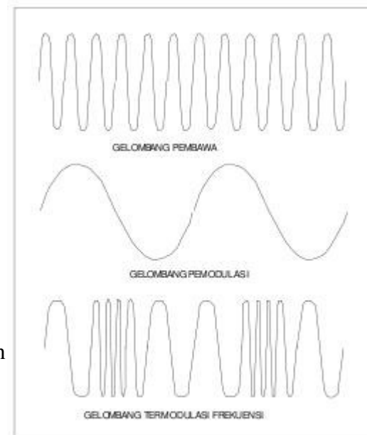
MODULASI FREKUENSI
