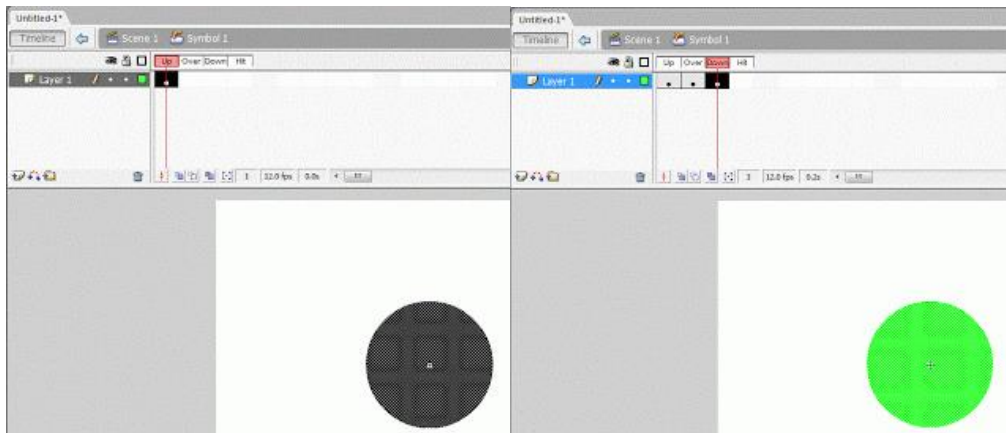
Gambar 121. Pengarah gambar
