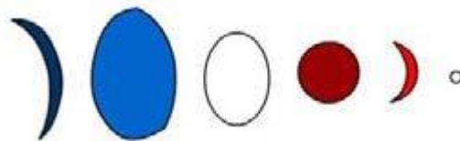
Gambar 55. Pemilihan warna
