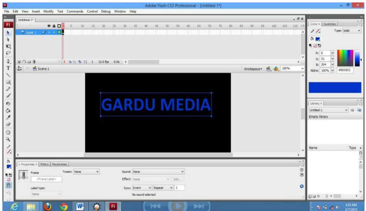
Gambar 14. Text Tool
