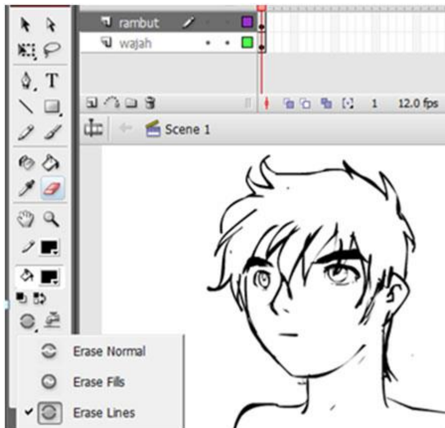
Gambar 98. Langkah 5
