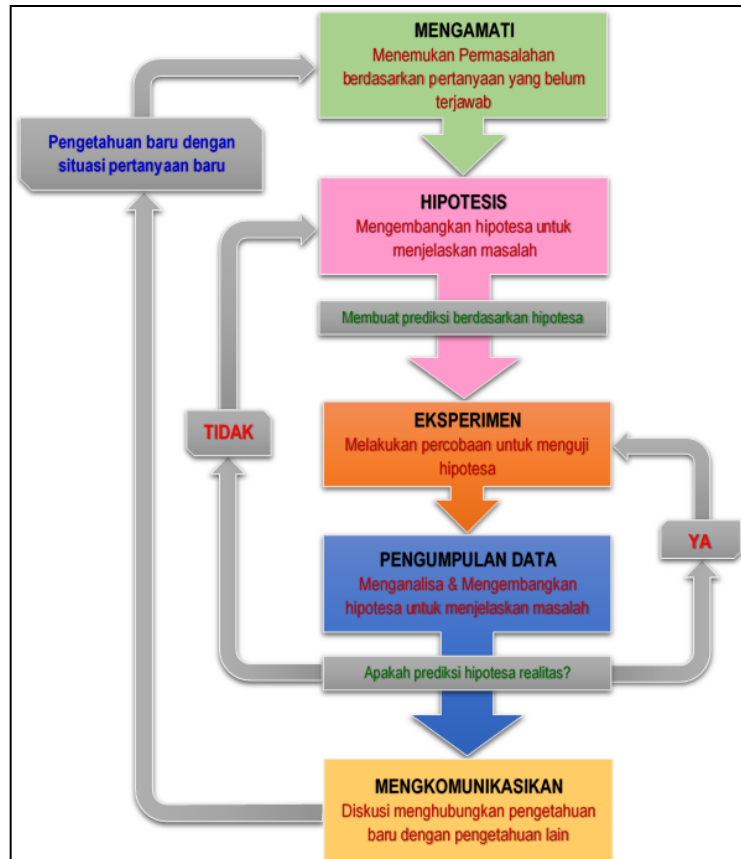
Gambar 3. Diagram Proses Metode Scientifik-Eksperimen Ilmiah
