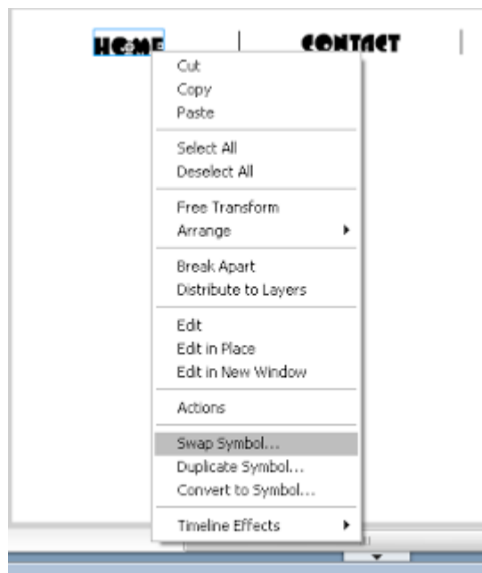
Gambar 140. Langkah selanjutnya
