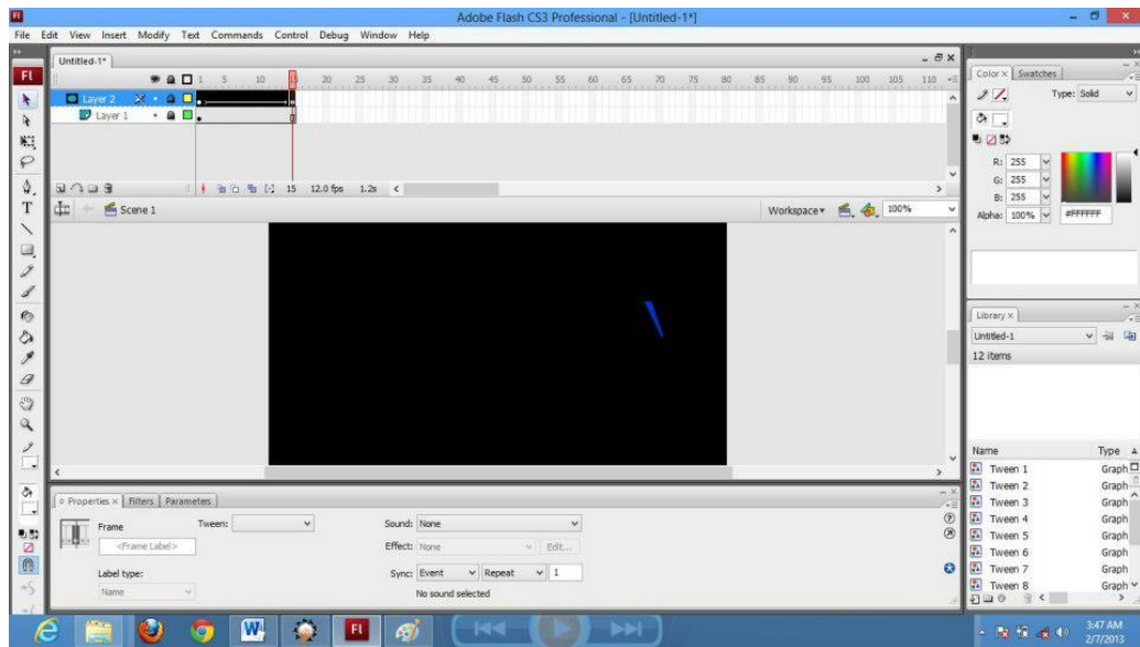
Gambar 19. Hasil masking
