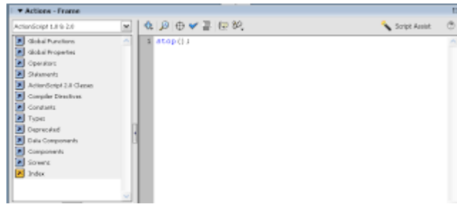
Gambar 132. Layer script
