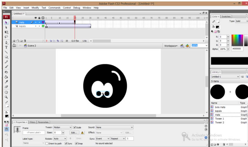
Gambar 174. Animasi bola
