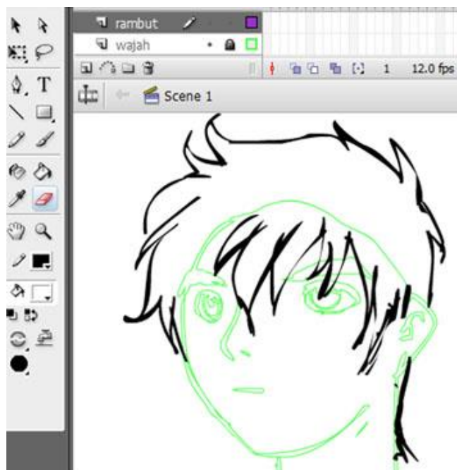
Gambar 110. Langkah 10
