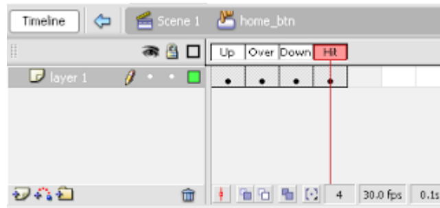
Gambar 139. Hasil Akhir
