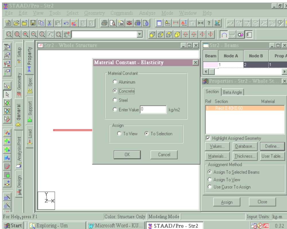
Gambar 2.29(b) Penentuan konstanta bahan struktur
